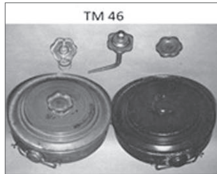
ภาพแสดงทุ่นระเบิดดักถถึงบางประเภทที่พบในประเทศไทย
