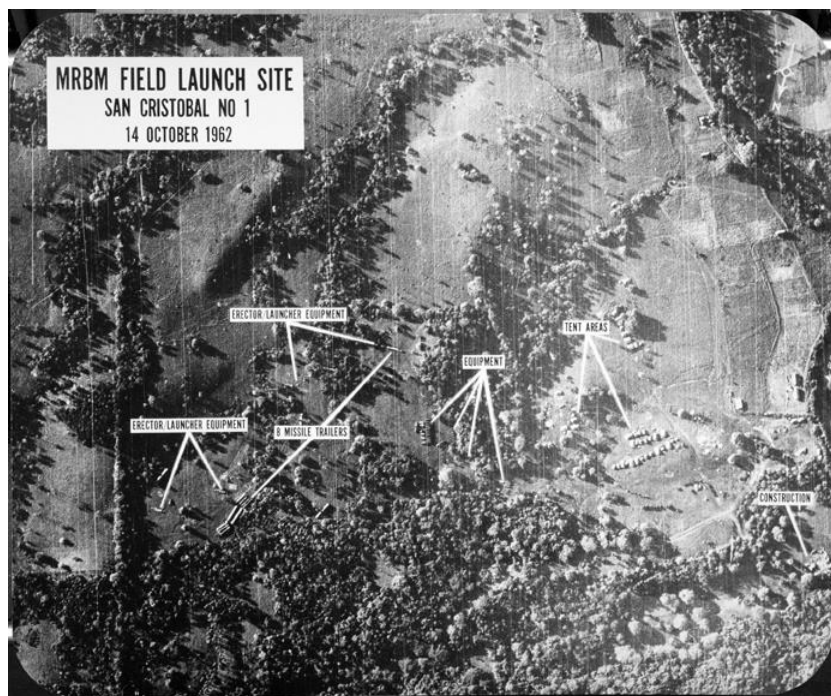
ภาพที่ 2 ฐานขีปนาวุธโซเวียตในคิวบากล่าวจากเครื่องบินสอดแนมของสหรัฐฯ 14 ตุลาคม ค.ศ. 1962
